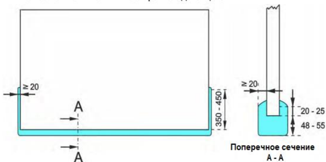
Рис. 8. Обивка щита
