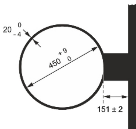
Рис. 5. Размеры баскетбольного кольца
