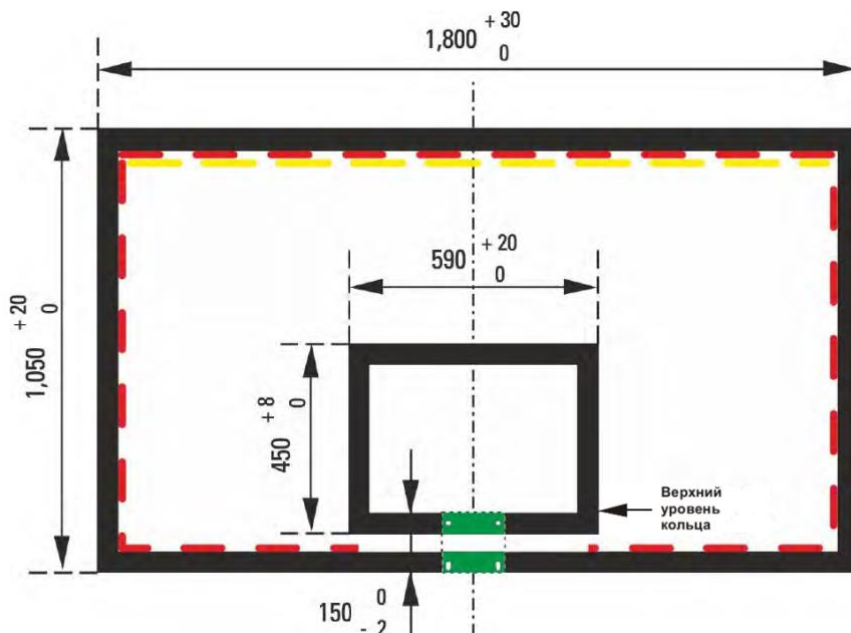
Рис. 3. Разметка щита
